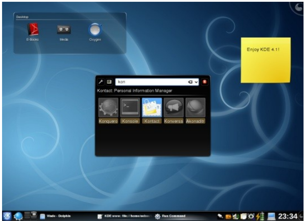
KDE Desktop
